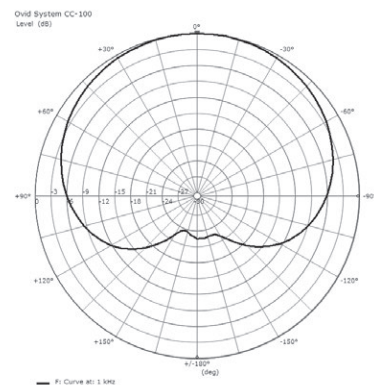
Polardiagramm @ 1 kHz
