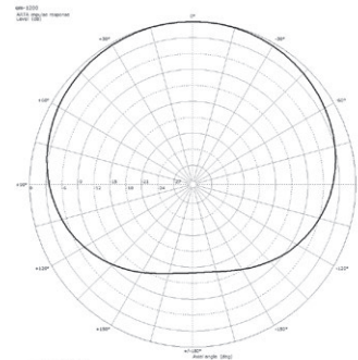
Polardiagramm @ 1 kHz
