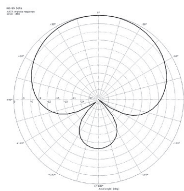
Polardiagramm @ 1 kHz
