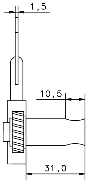
Seitenansicht von rechts side view rechts
