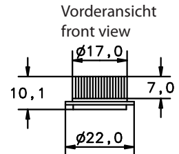
Gegenlager thrust bearing
