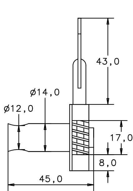
Seitenansicht von links side view left
